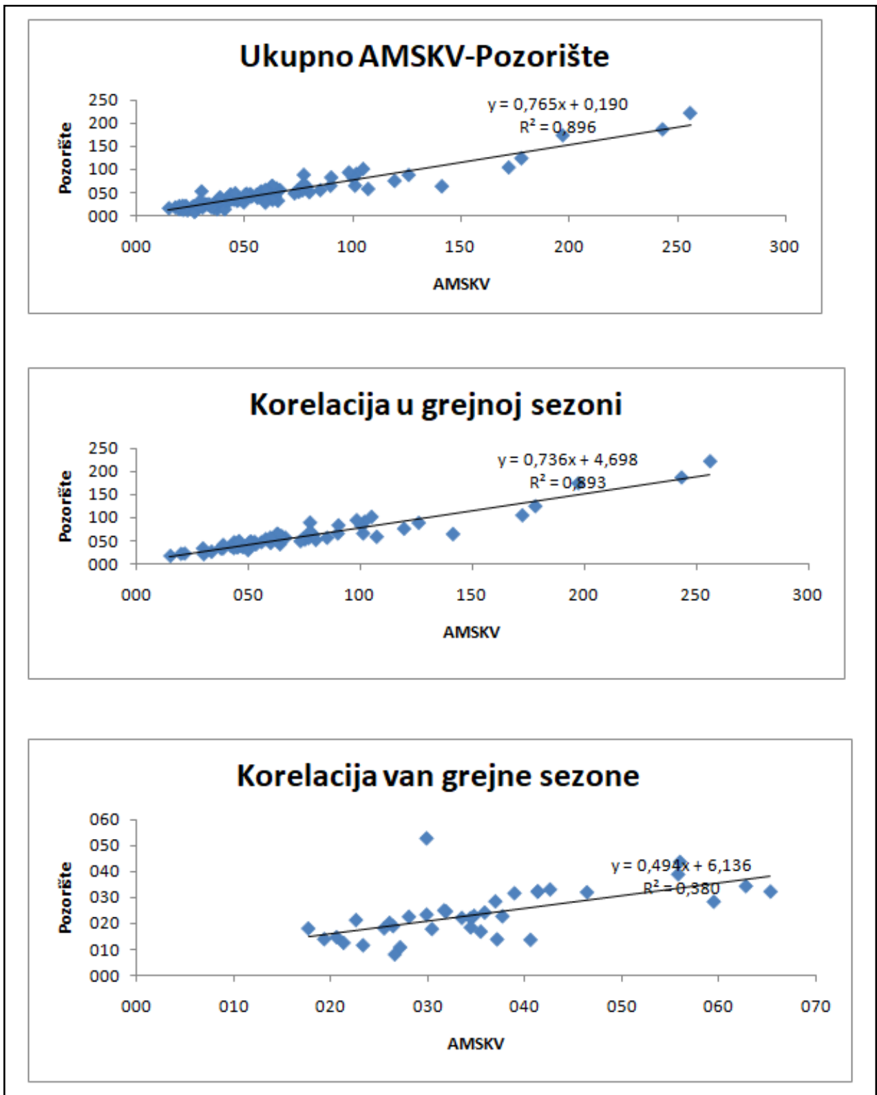
Слика бр.9: Упоредна анализа резултата концентрација суспендованих честица PM_{10} на мерним местима АМСКВ Ужице и Народно позориште Ужице
