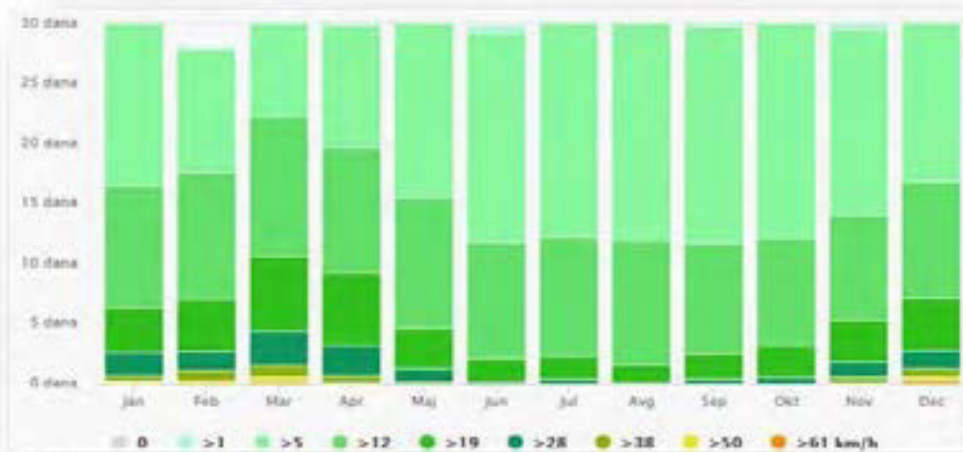
Графикон бр.5: Брзина ветра
