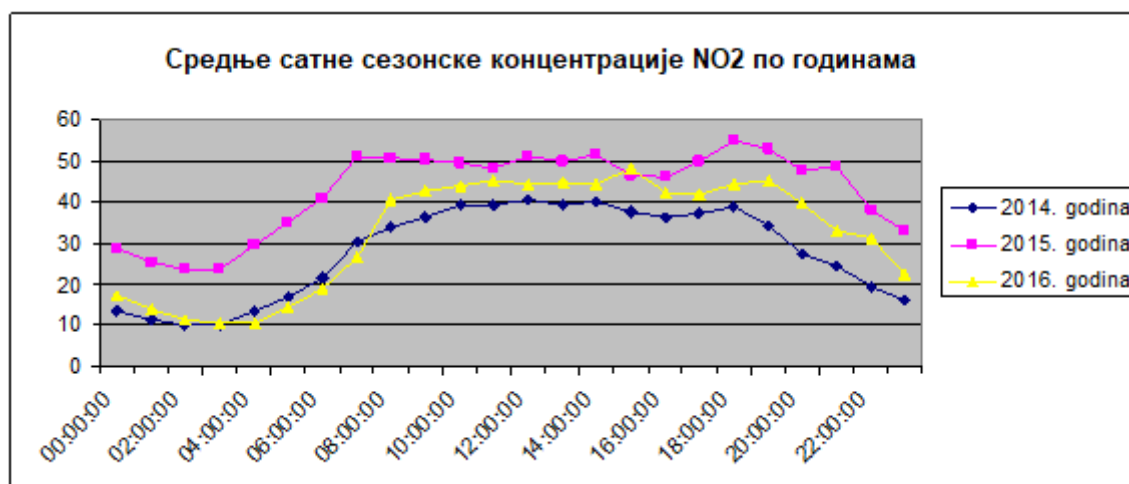
Графикон бр.11: Приказ средњих сатних концентрација \text{NO}_2 летњи период 2014-2016.год \mu\text{m}^3
