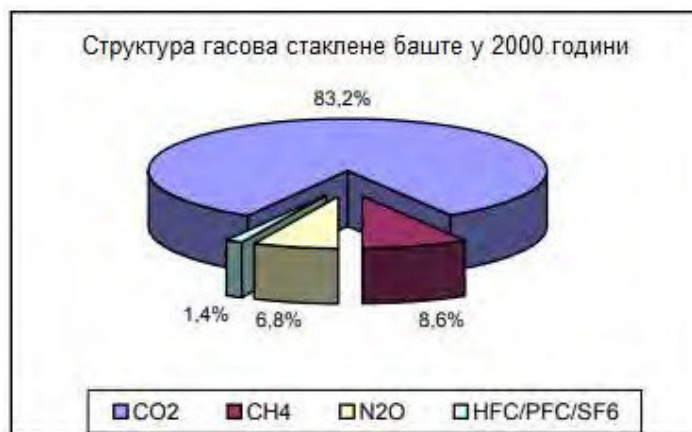
Слика бр.7: Структура гасова стаклене баште
