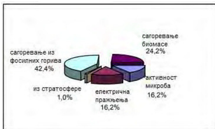
Слика бр.8: Структура порекла NOx
