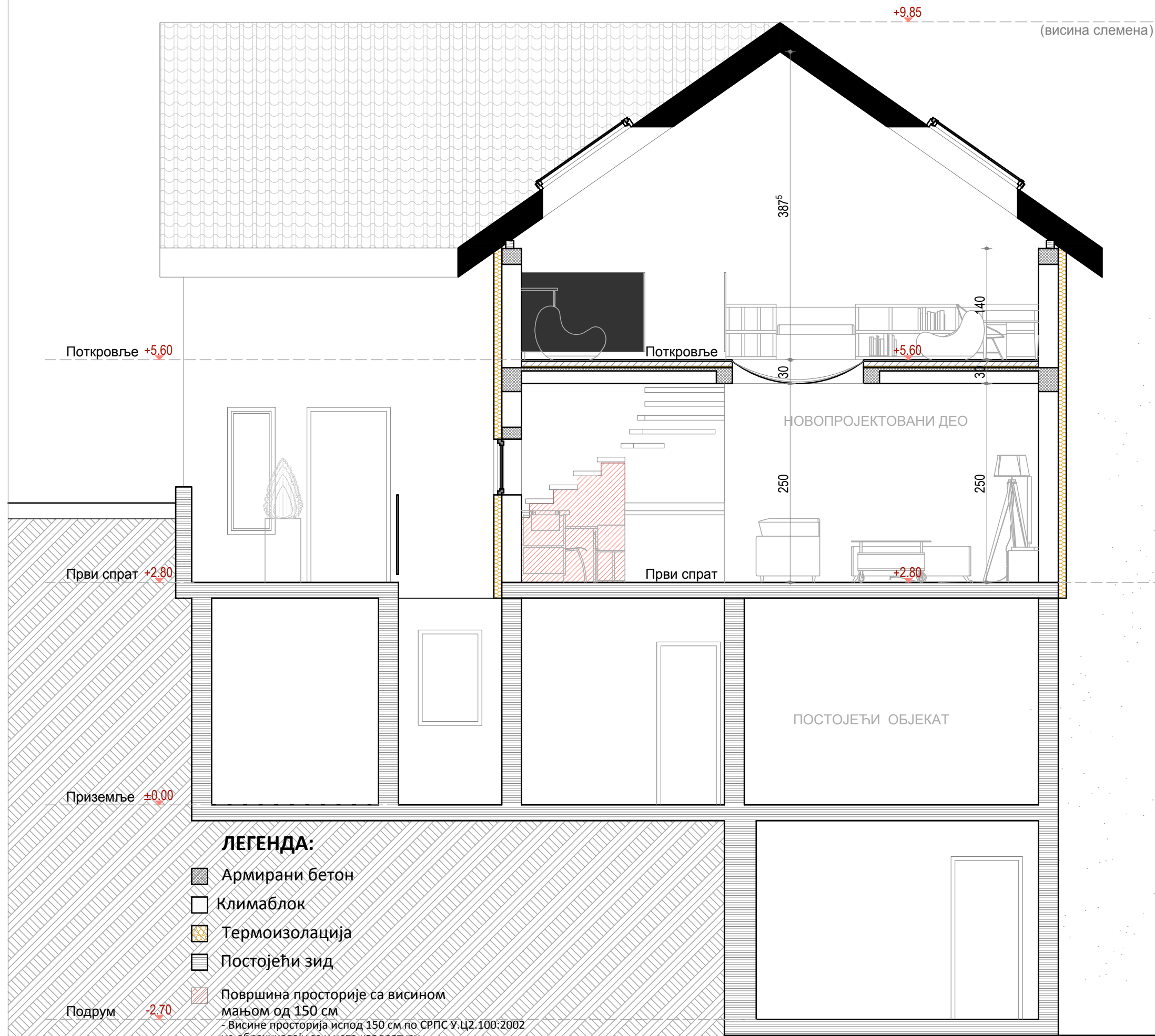
ПРЕСЕК А-А
