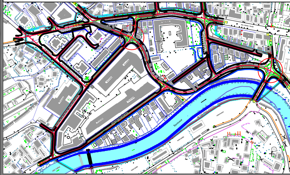
САОБРАЋАЈНО РЕШЕЊЕ- ФУНКЦИОНАЛНА ОРГАНИЗАЦИЈА - ФАЗА 1
