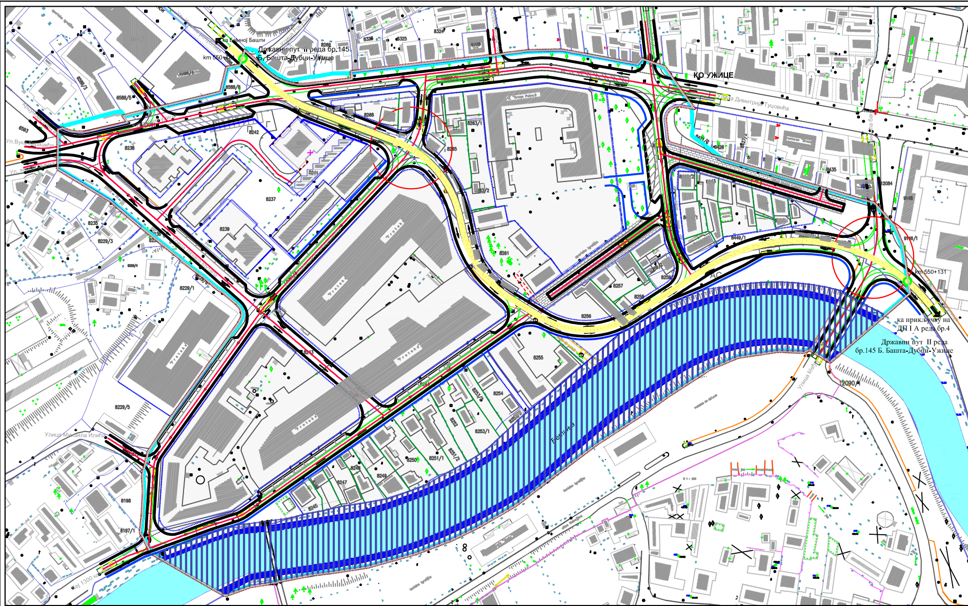
САОБРАЋАЈНО РЕШЕЊЕ- ФУНКЦИОНАЛНА ОРГАНИЗАЦИЈА - ФАЗА 1
